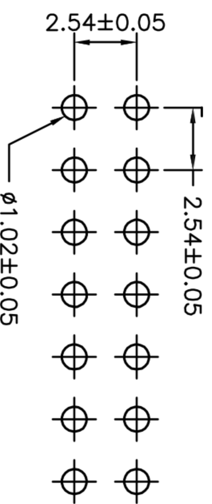
P.C.B. LAYOUT
