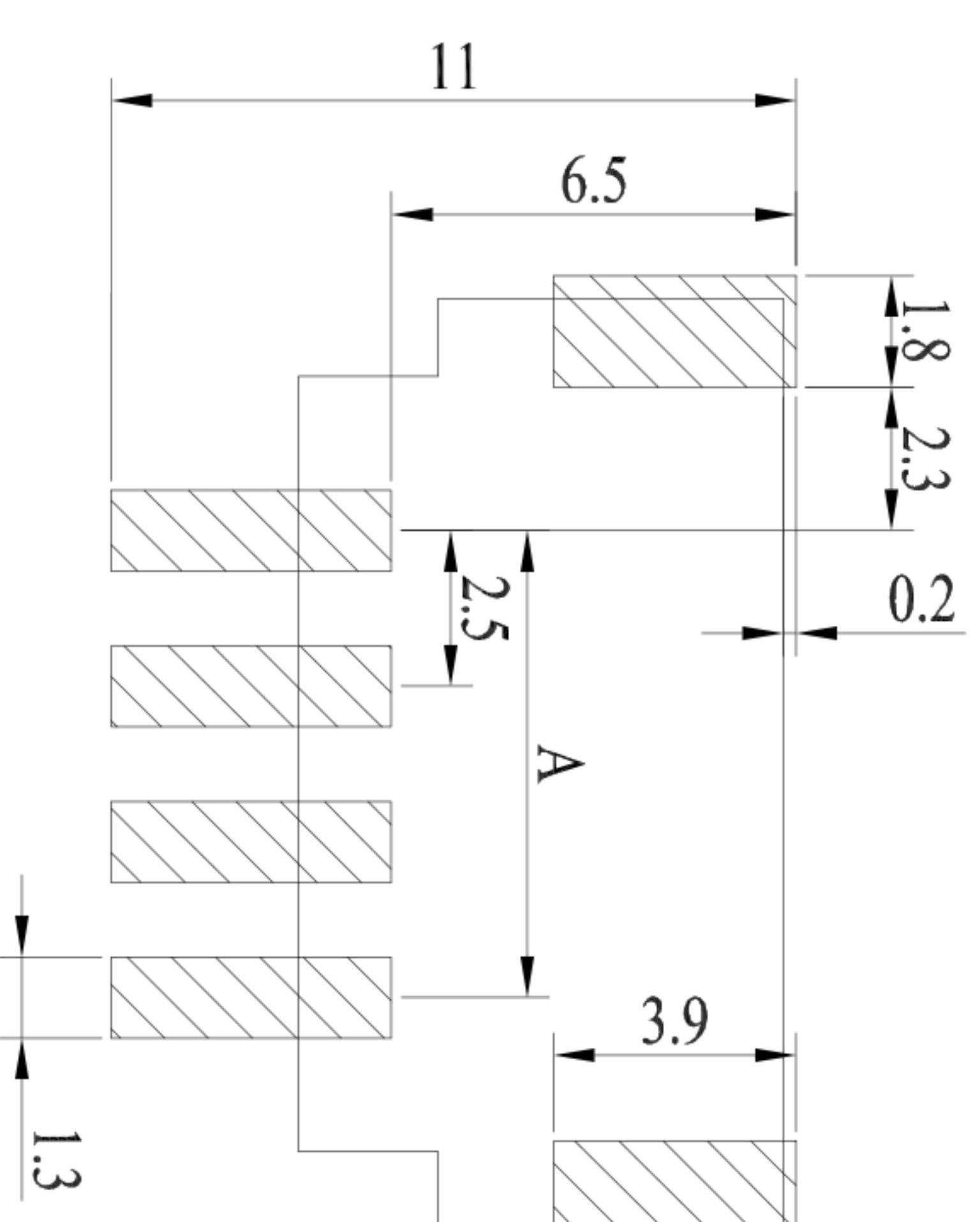
PCB板安装尺寸
